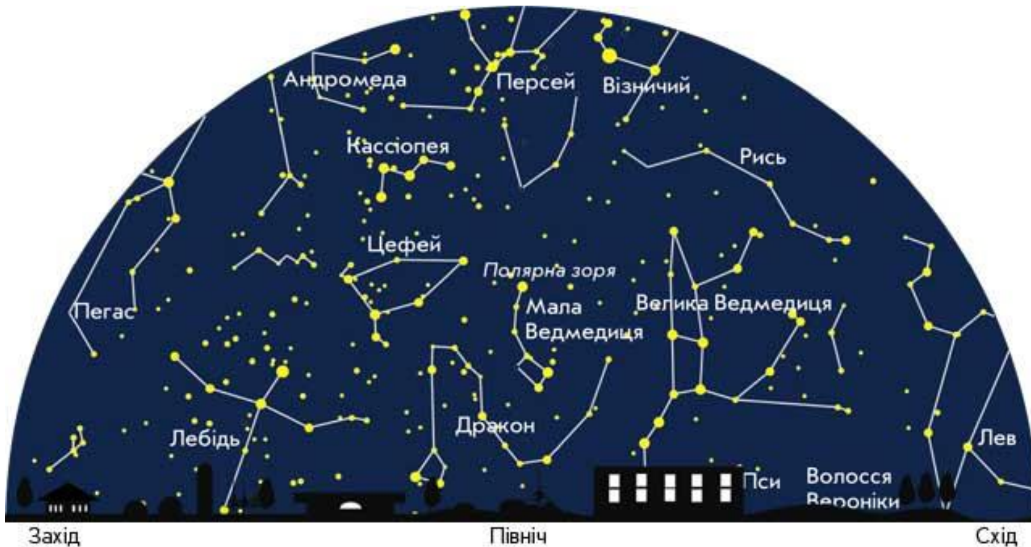
Вигляд північної частини зоряного неба в січні о 21 год київського часу на широті Києва
