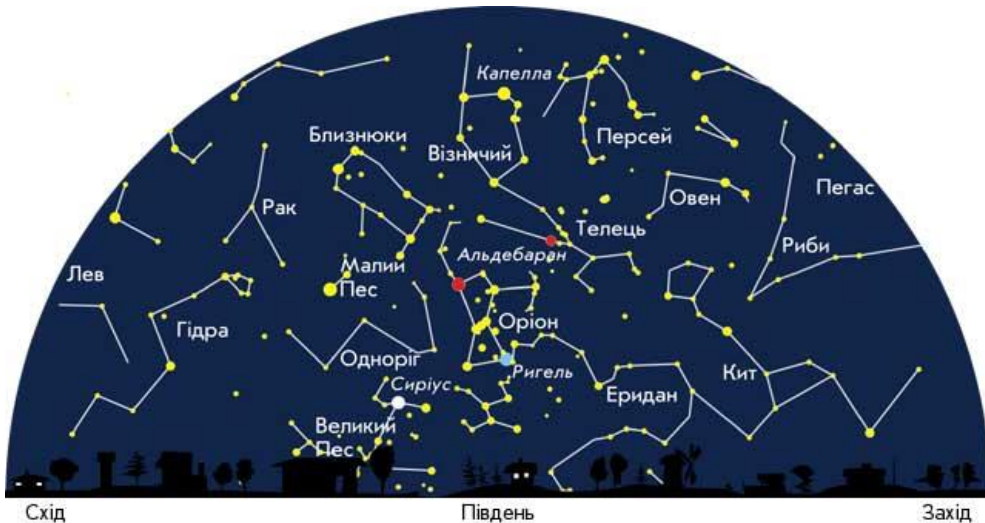
Вигляд південної частини зоряного неба в січні о 21 год київського часу на широті Києва
